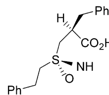
(2 S ,4 S )- 5
