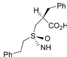
(2 S ,4 R )- 5
